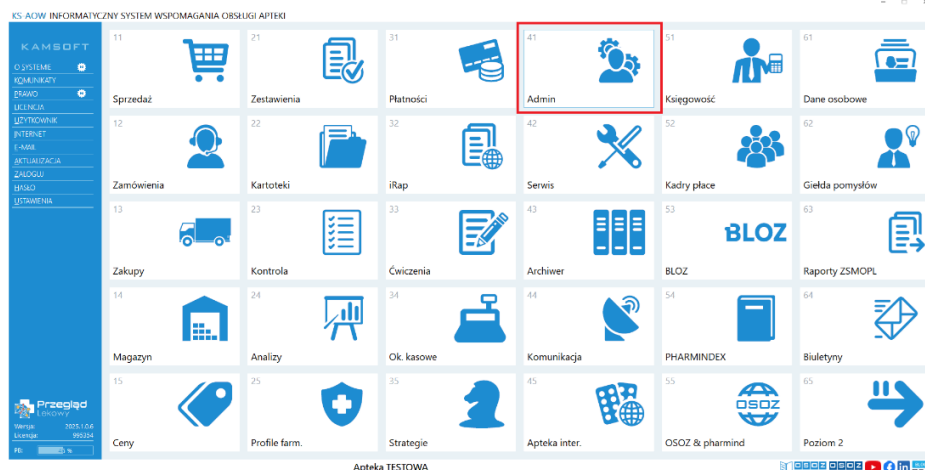
Rys. 7. Moduł APW41-Administrator
