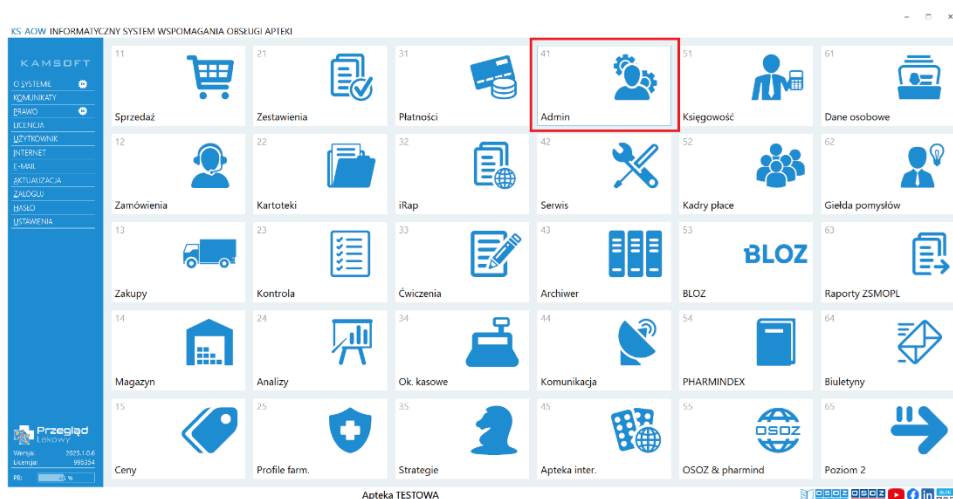
Rys. 2. Moduł APW41-Administrator.
