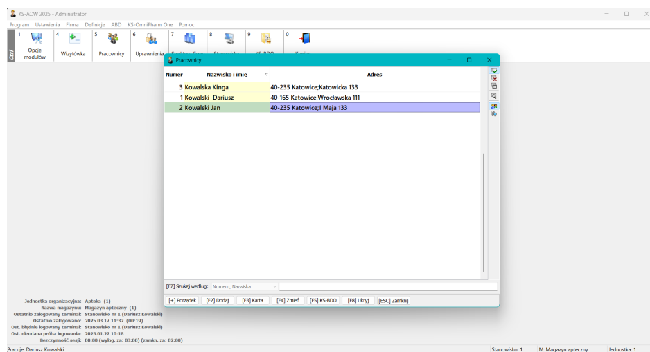
Rys. 4. Wybór pracownika.
