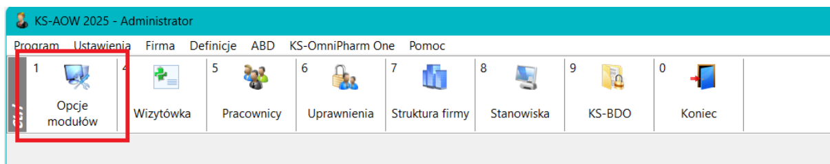
Rys. 8. Opcje modułów
